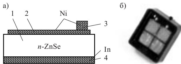
Рис. 1. Схематическое изображение (а) и внешний вид (б) УФ-фотодиода на основе ZnSe: 1 — кристалл ZnSe; 2 — полупрозрачный слой Ni; 3 — контактный слой Ni; 4 — омический контактный слой In
